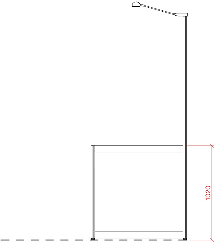
3 Elevation - Right A03 1 : 25
